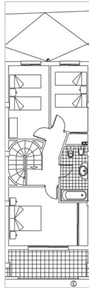
PLANTA SEGUNDA
